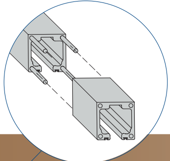
Bovenrail bevestiging Guide junction
